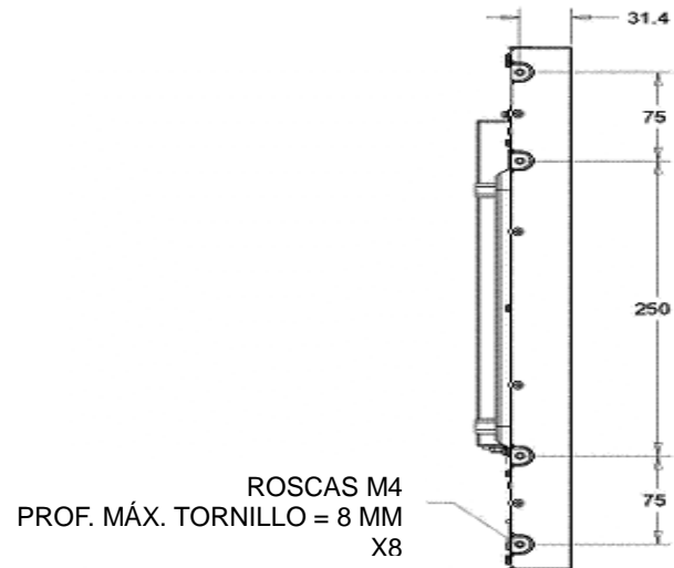
MONTAJE LATERAL VERTICAL (IZQUIERDA/DERECHA)
