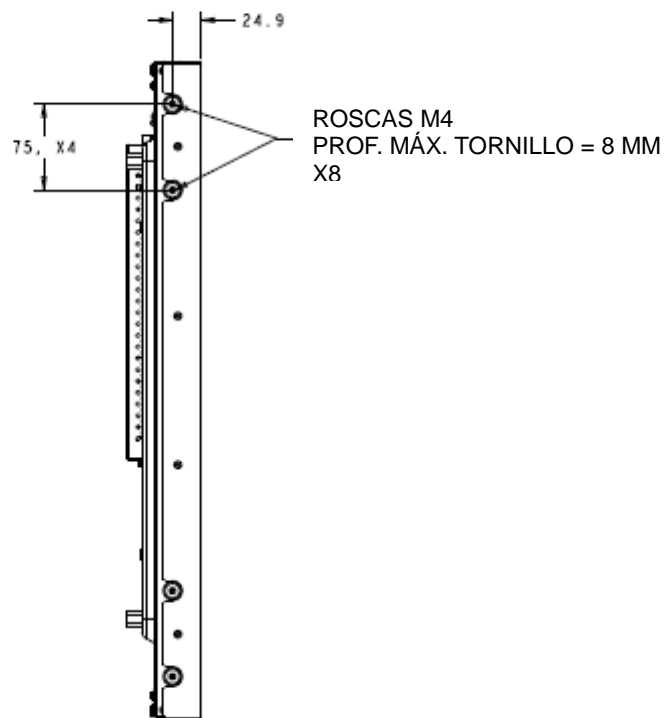
MONTAJE LATERAL VERTICAL (IZQUIERDA/DERECHA)
